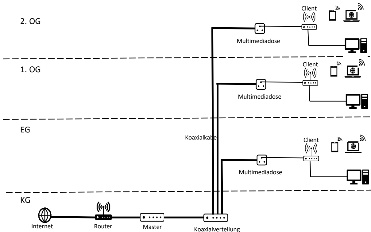
Abbildung 14: Koaxialnetzwerk
