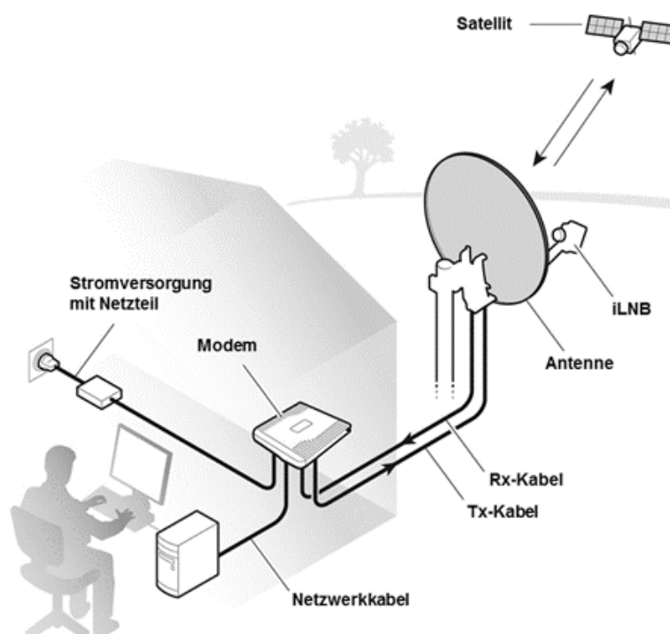
Abbildung 10: SAT-Internetanschluss
